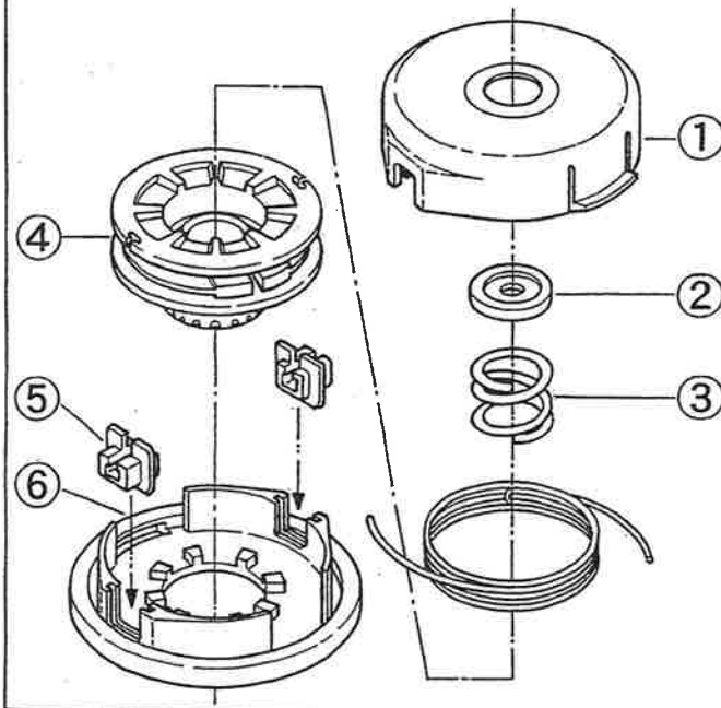
部品の名称
