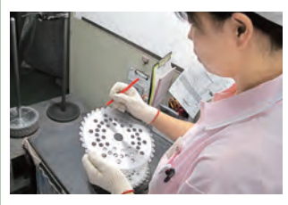
⑧ ろう付部の目視検査 (全数)
