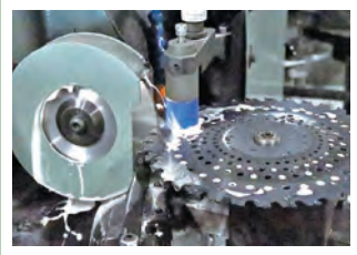
⑩ 超硬チップをダイヤ砥石で研磨
