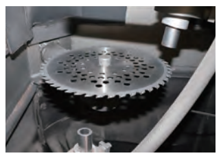
⑦ ショット加工
